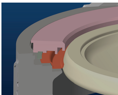
Уплотнение металл по металлу
