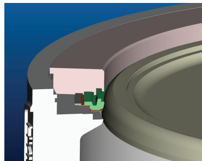
Uszczelnienie Fire safe
