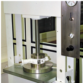
Испытания на герметичность и прочность сверхчистым азотом
